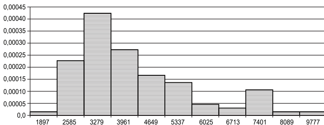
Рис. 1. Гістограма
