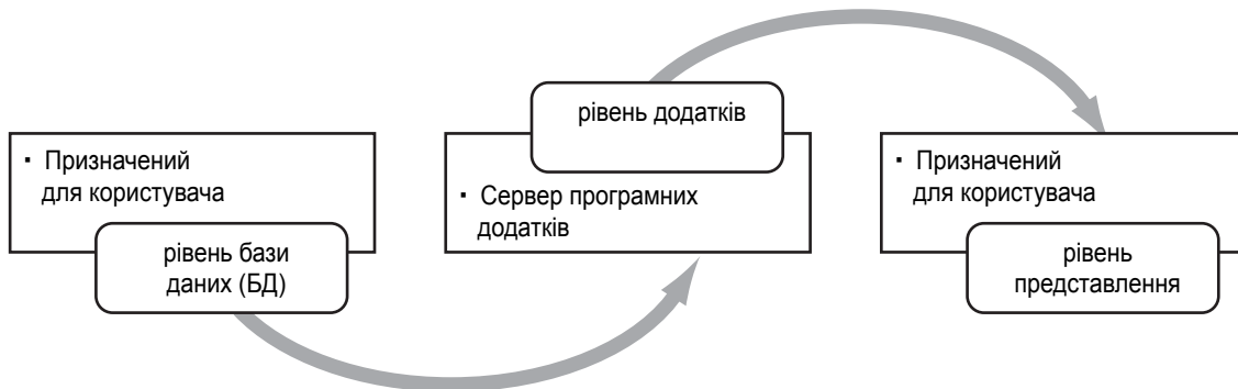
Рис. 1. Архітектура ERP-системи
