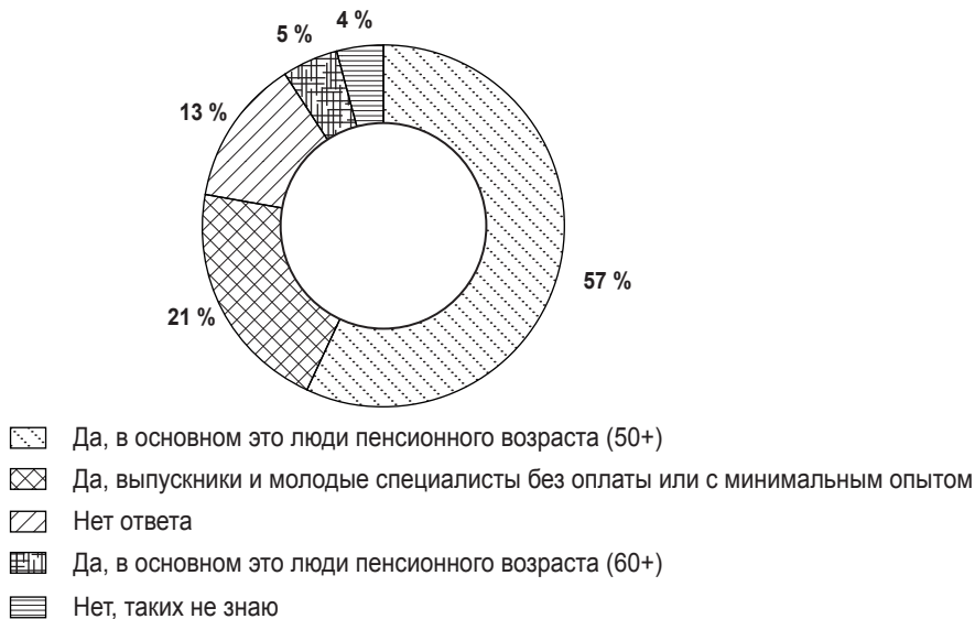
Рис. 1. Результаты опроса № 1
